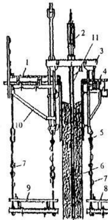
Рис.2 Скользящая опалубка
