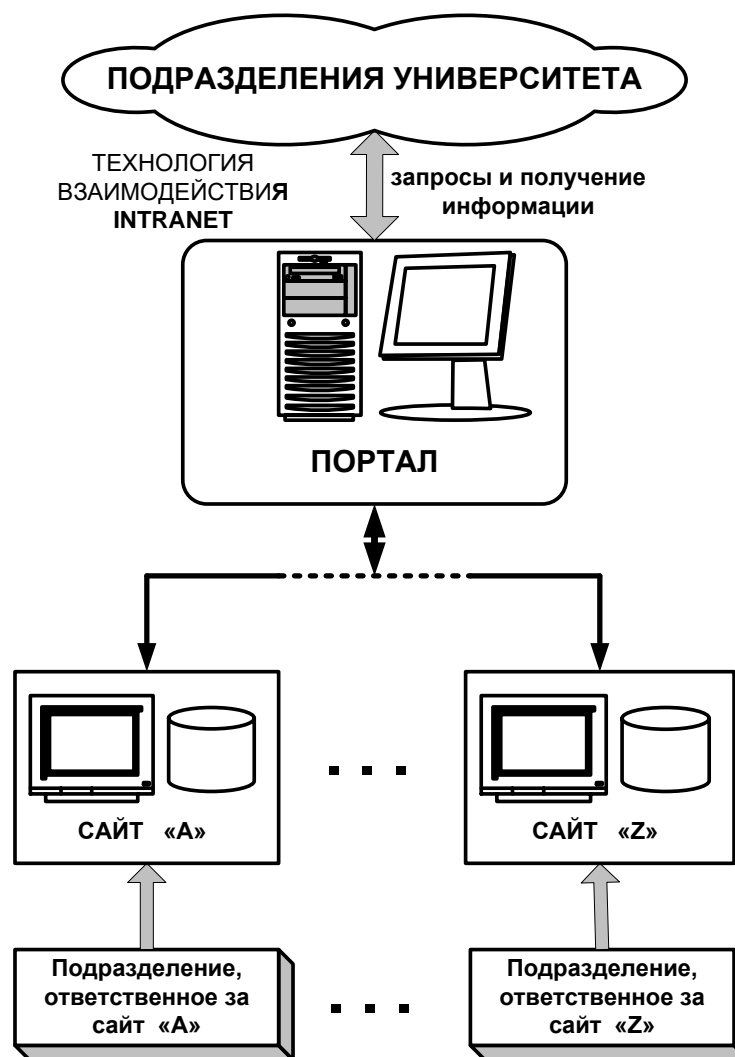
Рис.3. Структура информирующей системы
