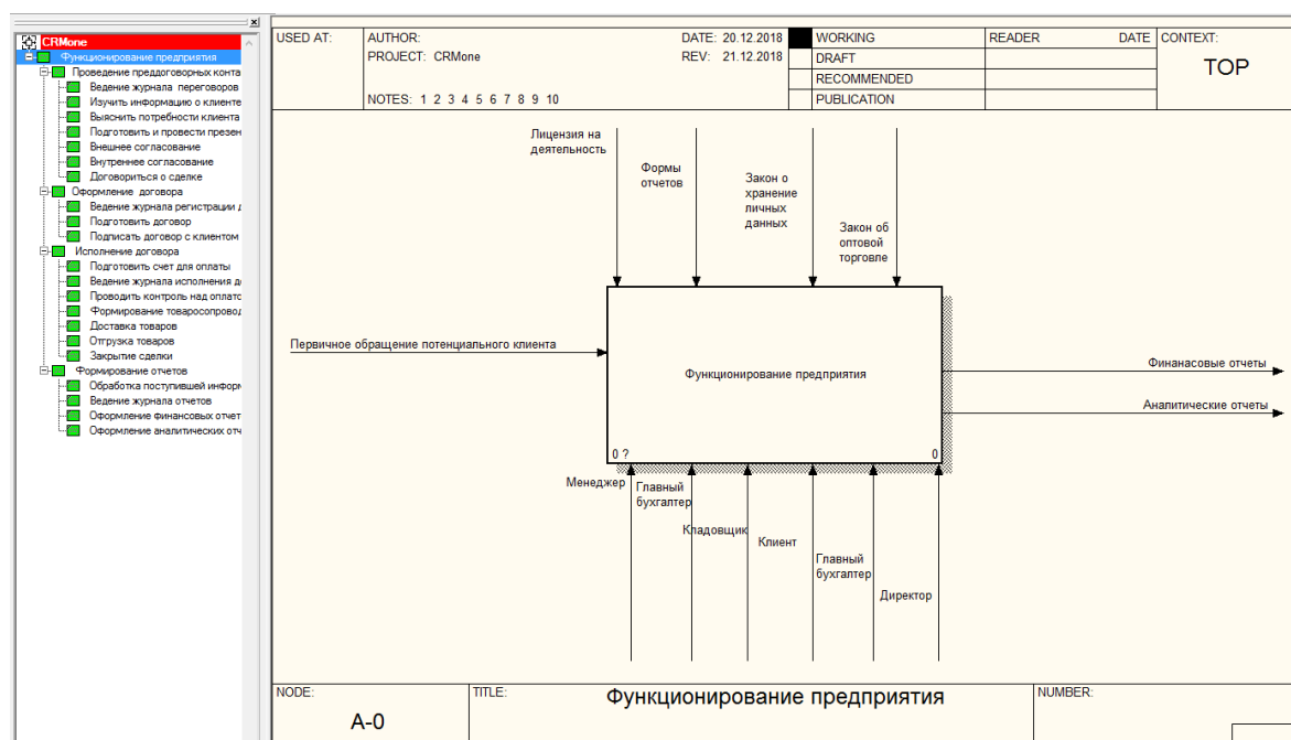
Рис. 1 – IDEF0. Контекстная диаграмма деятельности предприятия
