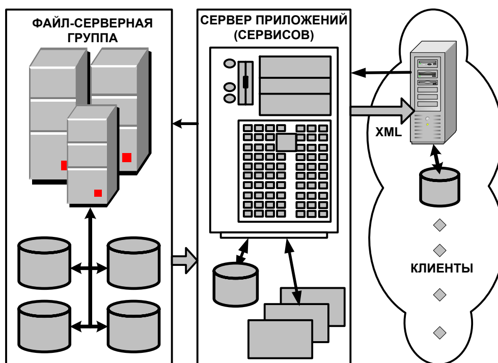
Рис. 5. Трехзвенная структура комплекса системных сервисов
