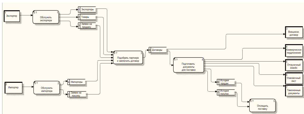
Рис. 3. Диаграмма потоков данных DFD
