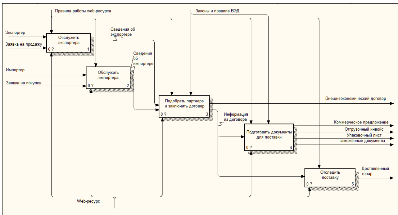
Рис. 1. Фрагмент диаграммы IDEF0
