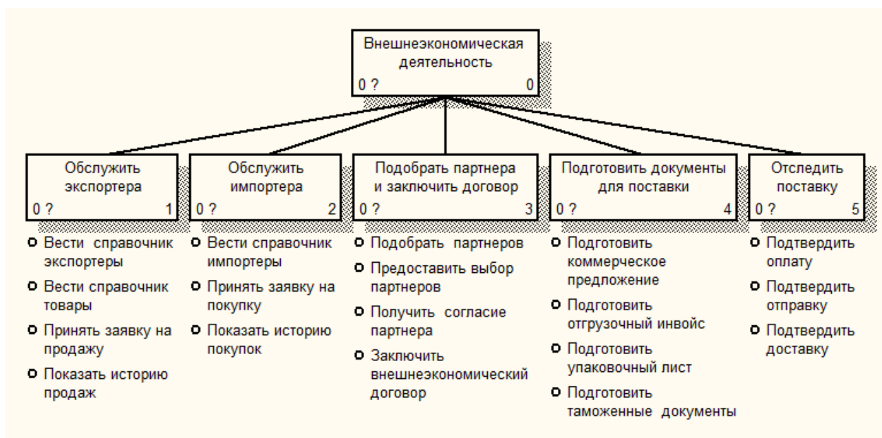
Рис. 2. Дерево узлов
