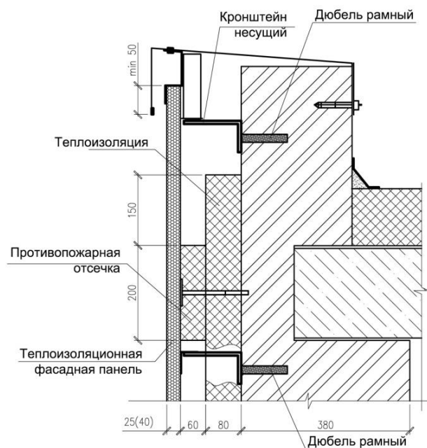
Рис. 1. Конструкция навесной системы «АЛПАН» при вертикальном расположении панелей.
