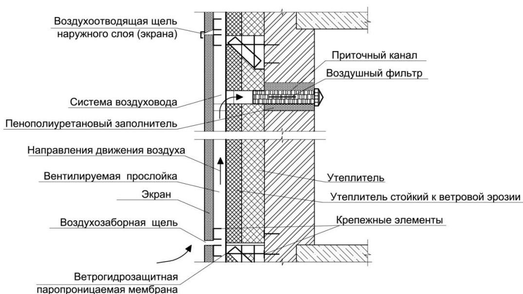
Рис. 2. Конструкция навесной системы «АЛПАН» преобразованная в ЭВОК.
