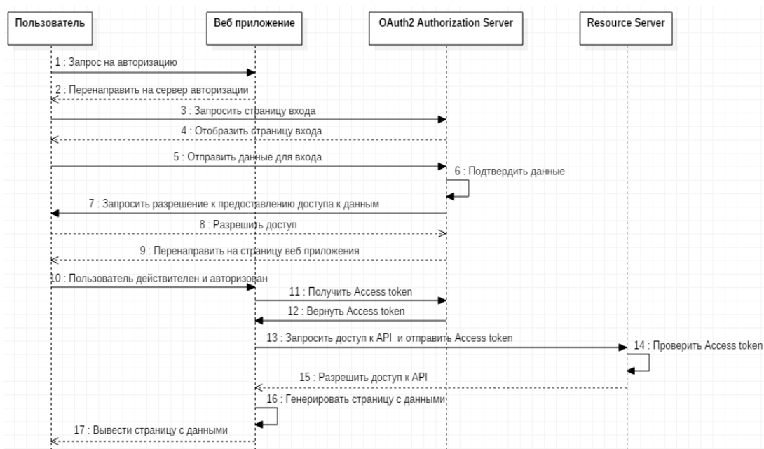
Рис. 1 Схема протокола OAuth 2.0
