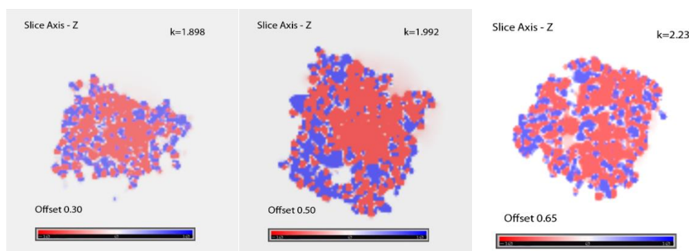
Рис. 3 – Проекционные срезы модели белка \beta -лактоглобулина в водной оболочкой, при значении рН=2
