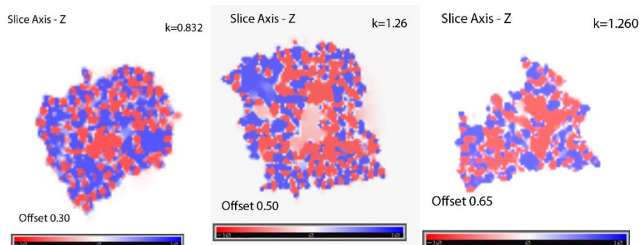
Рис. 4 – Проекционные срезы модели белка \beta -лактоглобулина в водной оболочкой, при значении рН=7
