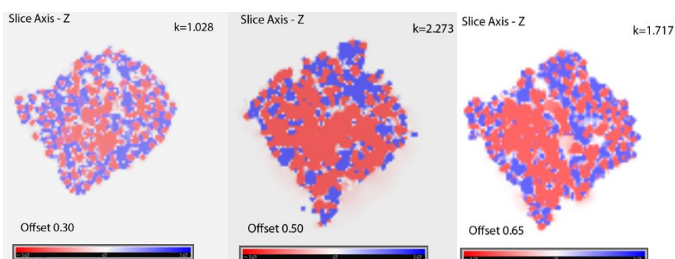
Рис. 5 – Проекционные срезы модели белка \beta -лактоглобулина в водной оболочкой, при значении рН=11
