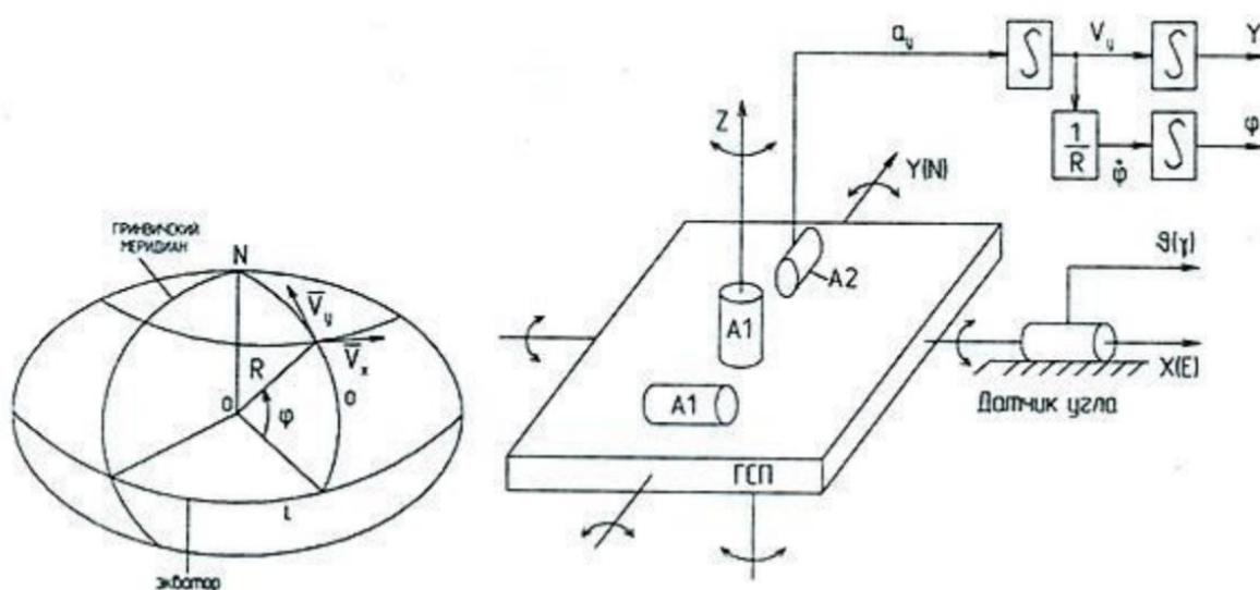
Рисунок 1 – Принцип построения ИНС
