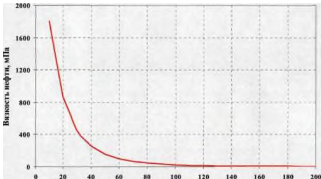
Рисунок 2 – Зависимость вязкости нефти от температуры Ван-Еганского месторождения, пласт ПК 1-2
