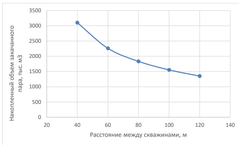
Рисунок 5 – График накопленного объема закачанного пара по вариантам
