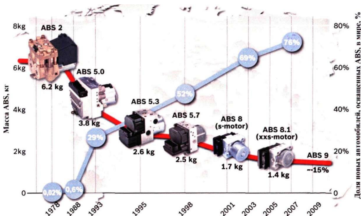
Рисунок 1.1- Динамика роста количества новых автомобилей, оснащенных ABS
