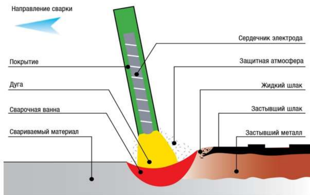
Рис. 1. Дуговая наплавка.
