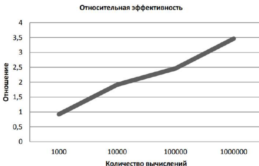
Рис. 2. Относительная эффективность многопоточных и однопоточных приложений.
