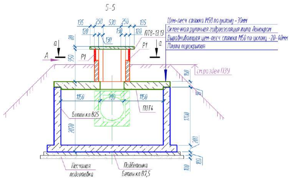
Рис.5. Вентиляционная шахта в монолитном канале.
