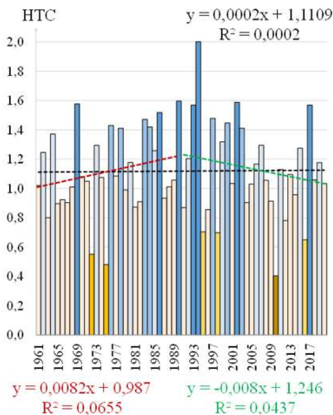
Рис. 2. Временное распределение гидротермического коэффициента Селянинова в Республике Башкортостан за 1961-2020 гг.
