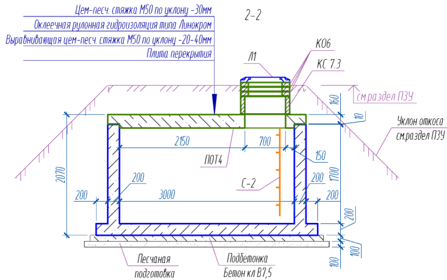
Рис.6. Опуск в монолитный канал.
