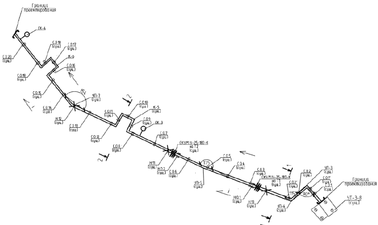
Рис.3. Монтажная схема тепловой сети.
