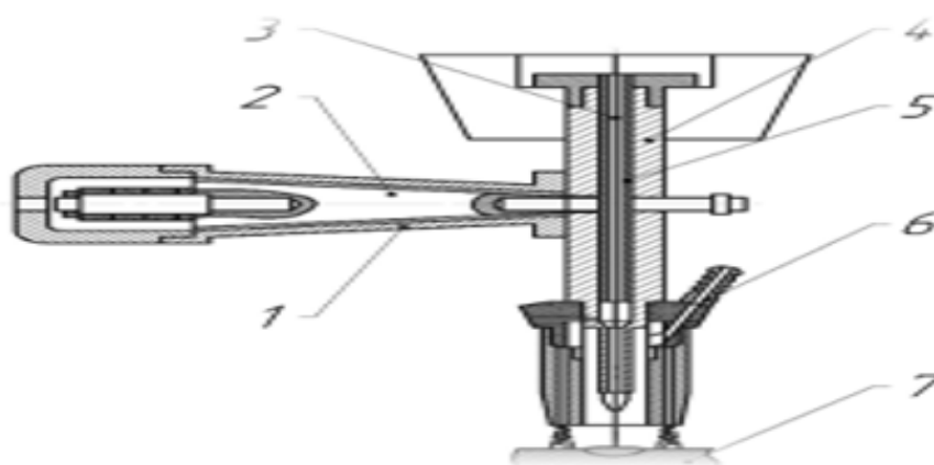
Рис. 3. Схема технологической установки для наплавки с ультразвуком и металлопорошковой присадкой:
