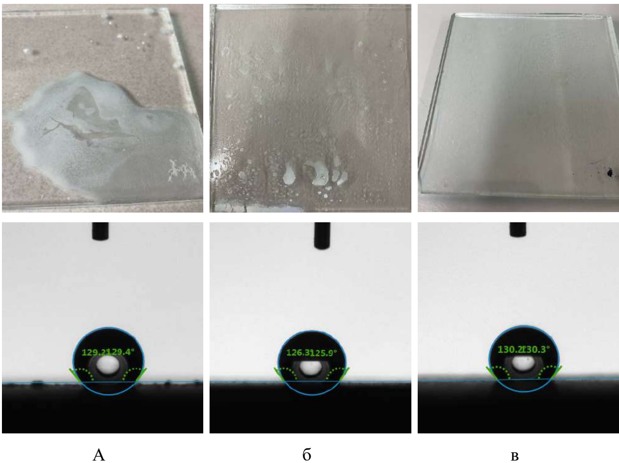
Рис. 2. Внешний вид и контактный угол смачивания образцов поверхности стекла, обработанных растворами: а – Neomid H2O Stop, б – Полипласт Барьер 203, в – Типром К Люкс,
