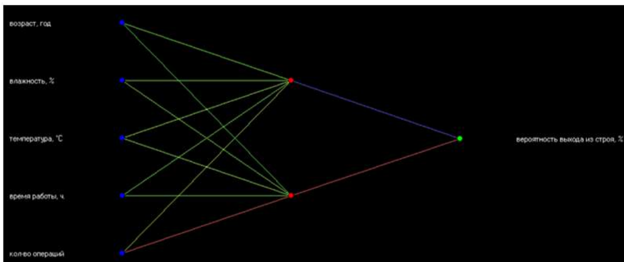
Рис. 1. Граф нейросети.
