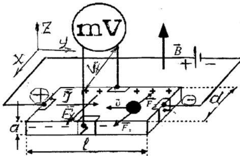
Рис 1. Схема эксперимента Э.Холла.
