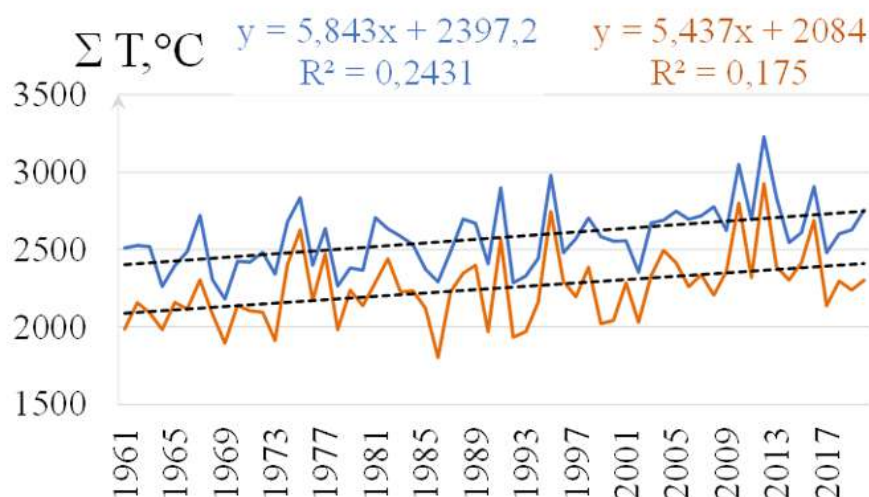
Рис. 1. Многолетний ход \Sigma T \geq 0 °С и \Sigma T \geq 10 °С, осредненных в Республике Башкортостан за 1961-2020 гг.
