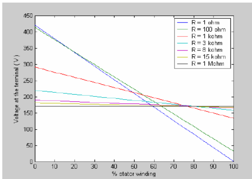
Рис.5. Третьи гармоники напряжения на выводах обмотки.
