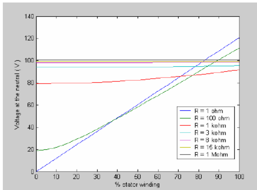
Рис.4. Третьи гармоники напряжения со стороны нейтрали.
