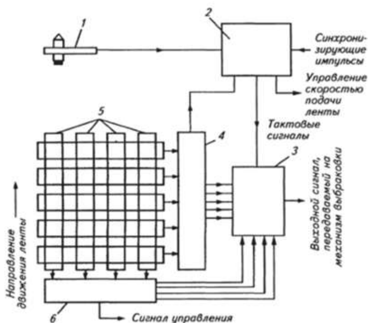
Рис. 2. Схема установки для полуавтоматической сортировки яиц: 1 - жезл; 2 - схема управления; 3 - регистровая память; 4 - дешифраторы поперечных рядов; 5 - матрицы; 6 - дешифраторы продольных рядов.
