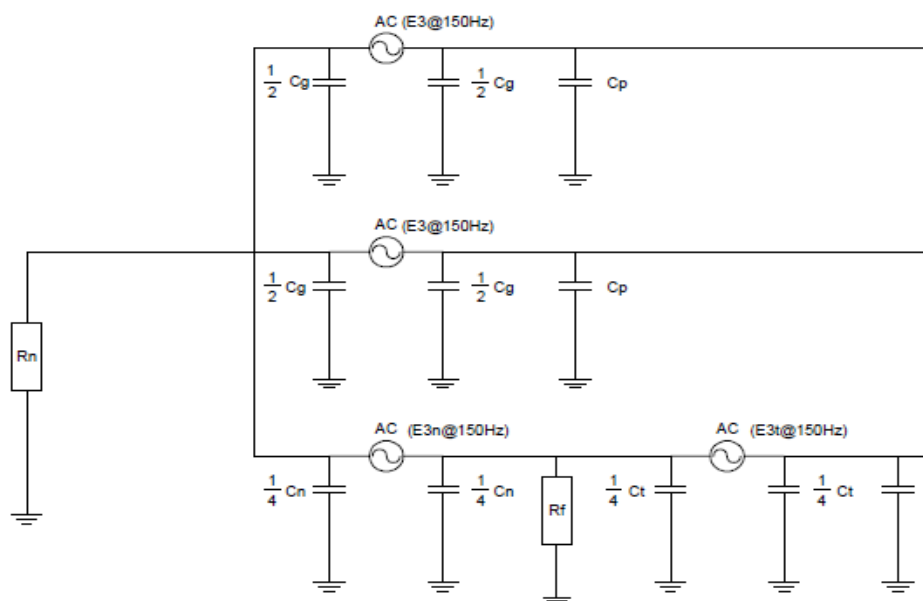
Рис.2. Эквивалентная схема замещения генератора в режиме замыкания.
