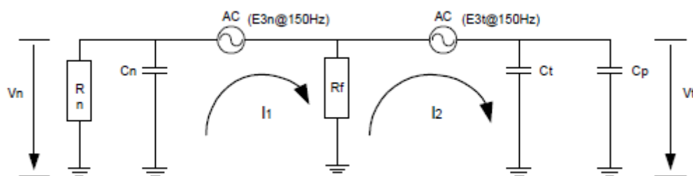
Рис.3. Схема замещения замыкания фазы на землю.
