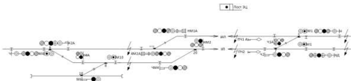
Рис. 1. Фрагмент схематического плана станции «К».
