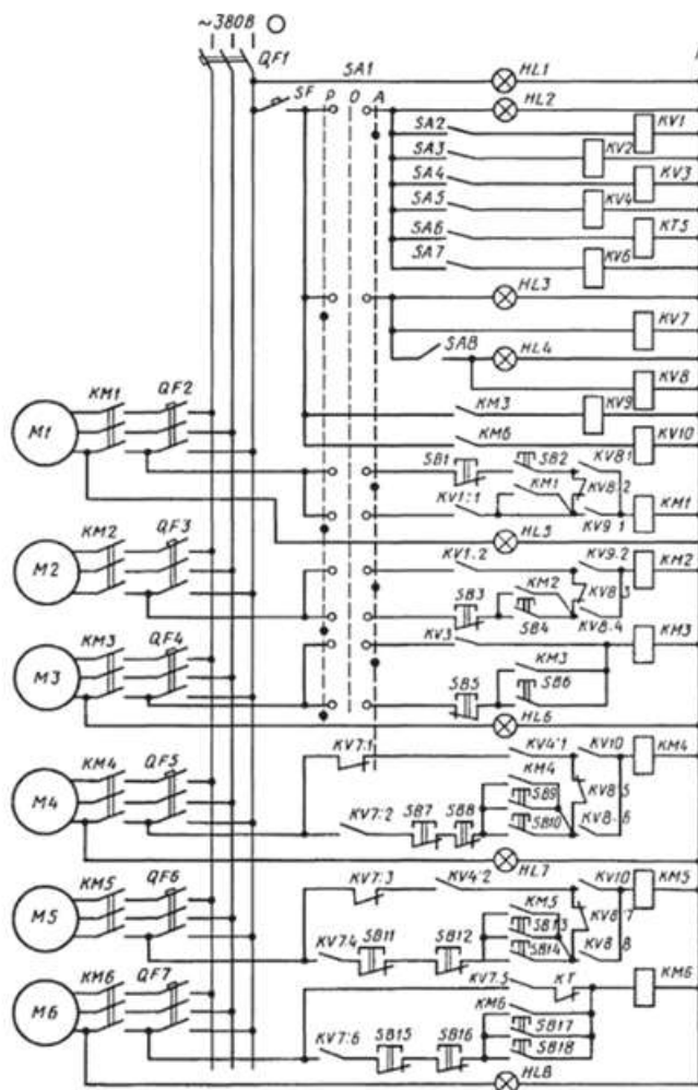
Рис. 1. Принципиальная электрическая схема управления сбора яиц с многоярусных клеток в птичниках
