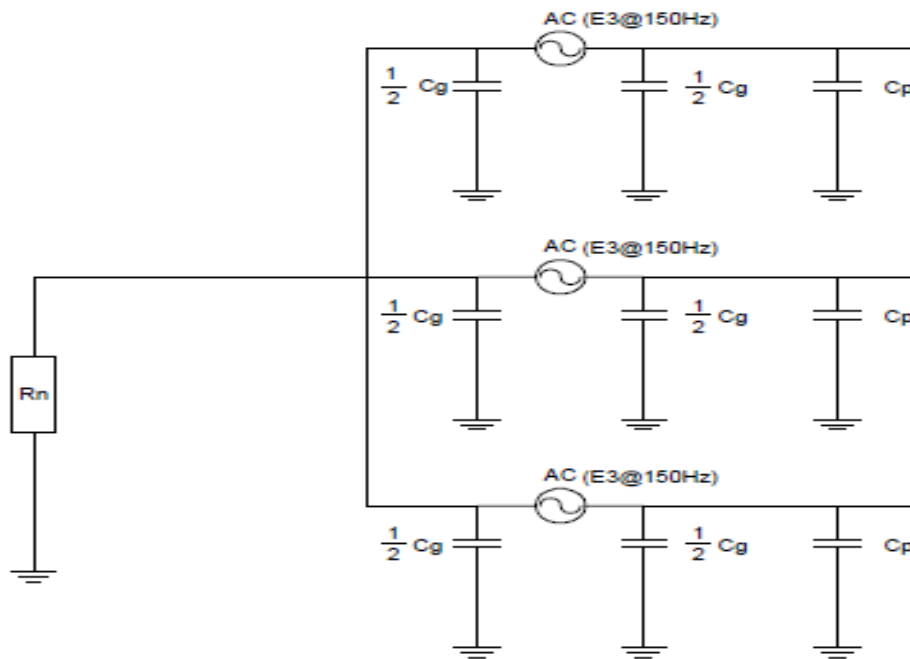
Рис.1. Эквивалентная схема замещения генератора в нормальном режиме.
