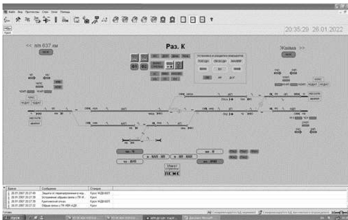
Рис. 2. Изначальная схема станции типа разъездная К в системе АДК СЦБ.
