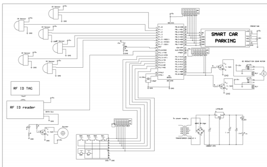
Рисунок 2. Система управления парковкой.
