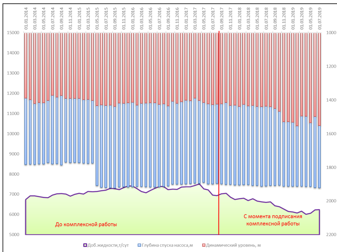
Рисунок 3 – Динамика основных среднесуточных показателей разработки. Объект БВ1-2 В период с 2017-2019 гг. в связи с ростом обводненности добываемой продукции
