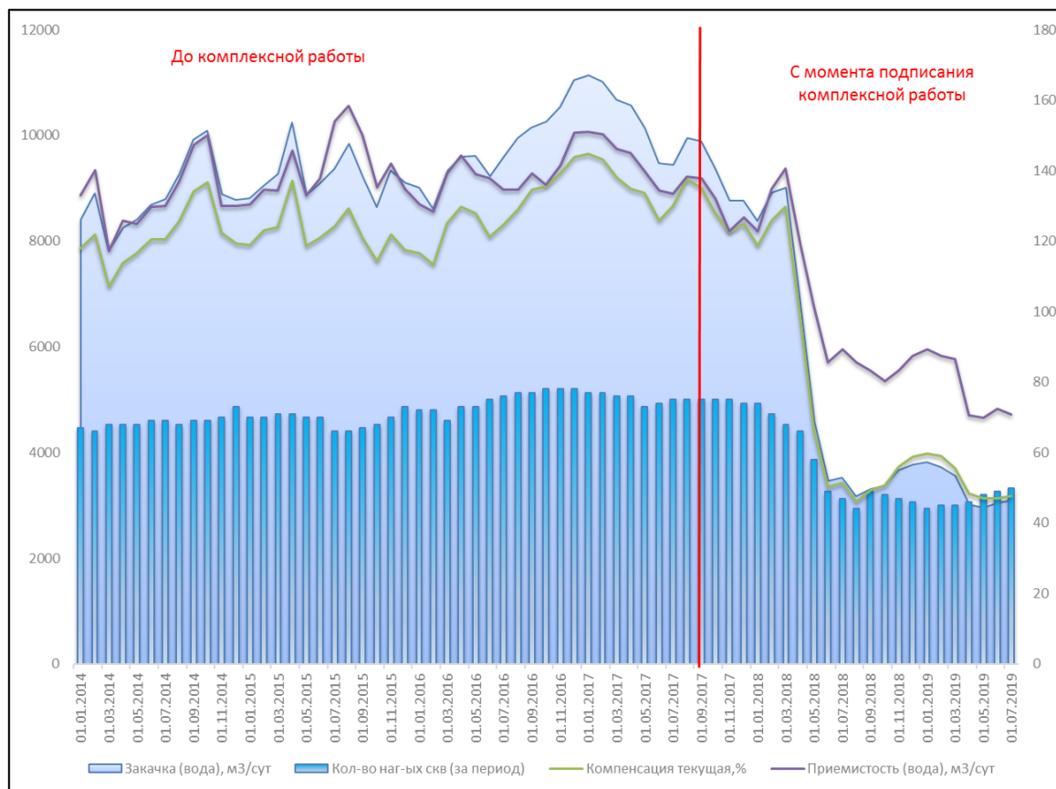
Рисунок 6 – Динамика нагнетательного фонда. Объект БВ 1-2
