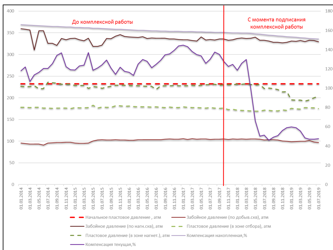
Рисунок 4 – Динамика изменения пластового давления и компенсации. Объект БВ 1-2
