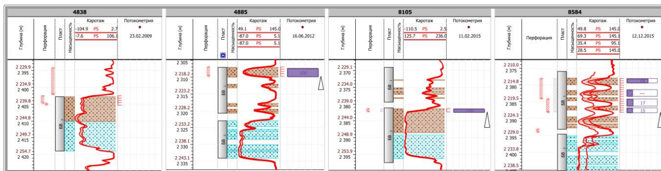
Рисунок 2 – Разрез и результаты потокометрии. Скважины 4838, 4885, 8105, 8584
