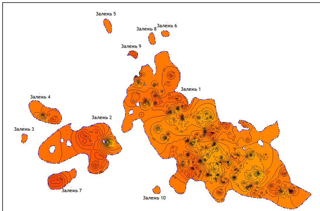
Рисунок 5 – Карта изобар по состоянию на 01.07.2019 г. Объект БВ 1-2
