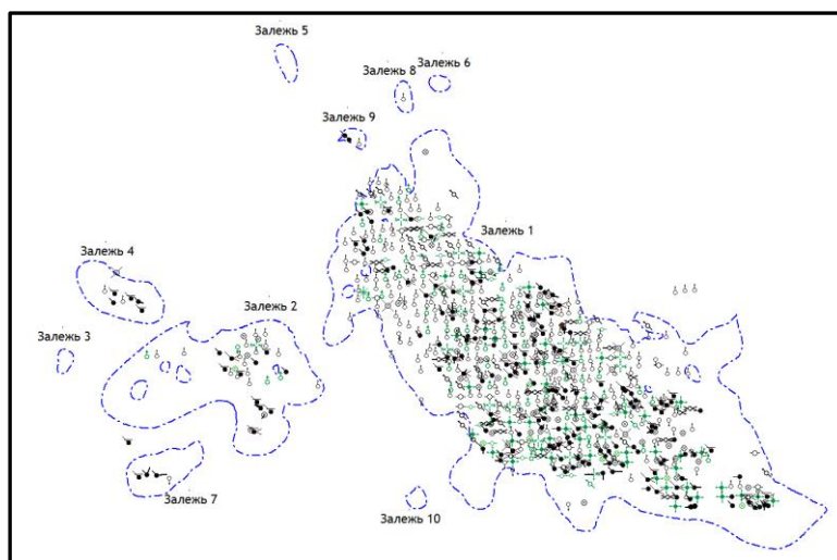
Рисунок 2 – Схема расположения скважин на Объекте БВ 1-2 Ватьеганского месторождения.
