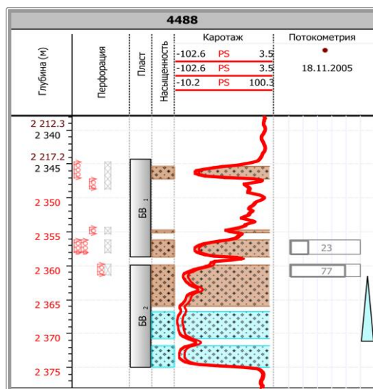
Рисунок 1 – Разрез и результаты потокометрии. Скважина 4488
