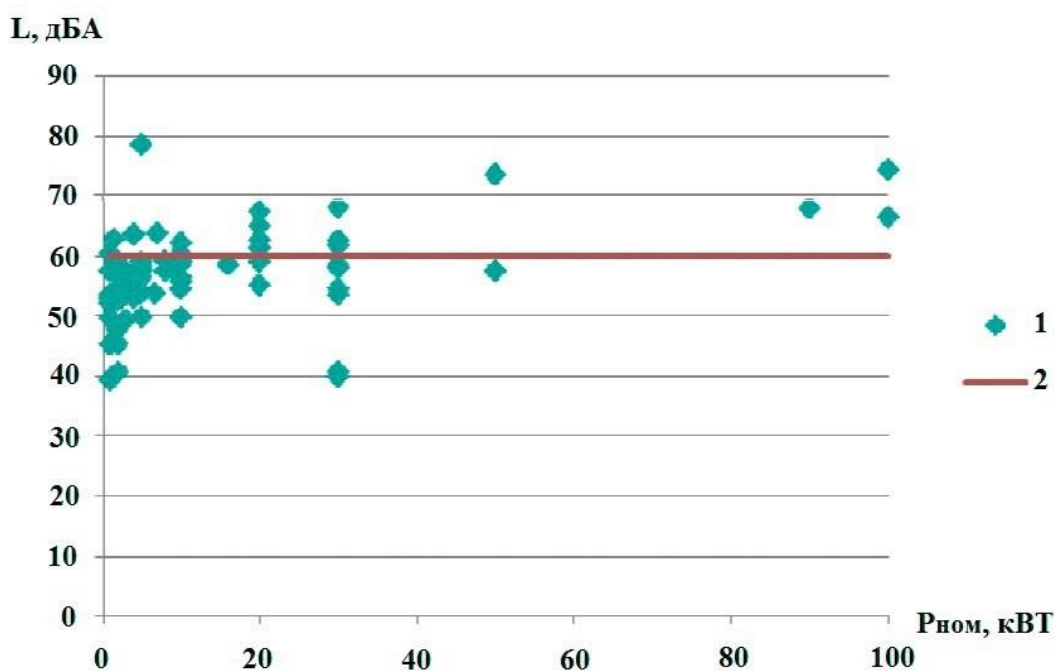
Рис. 1. Зависимость номинальной мощности ВЭУ P_{\text{ном}} (кВт) от уровня шума L (дБА) на расстоянии 50 метров от ВЭУ: 1 – шум от ВЭУ; 2 - допустимый уровень шума
