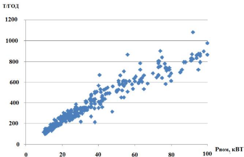
Рис. 2. Зависимость номинальной мощности ДГУ P_{ном} (кВт) от приведенной массы годового выброса загрязняющих веществ в атмосферу (т/год)
