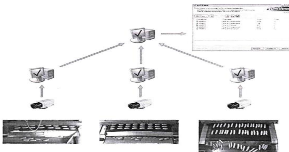
Рисунок 3. Структурная схема программно-технического комплекса оптического контроля количества продукции
