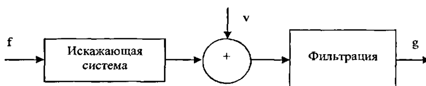
Рисунок 4. Структурная схема модели наблюдения полезного сигнала с последующей предобработкой: f - входное изображение, v - шумовая составляющая, g - выходное изображение.
