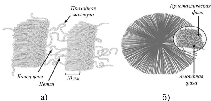
Рис. 2. Элементы надмолекулярной структуры частично – кристаллического полимера: а – ламели; б – сферолит.
