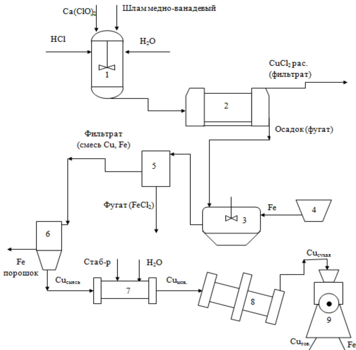
Рис. 1. 1 – Реактор с мешалкой; 2 – барабанный фильтр; 3 – Электролизер (восстановитель) или цементатор; 4 – бункер; 5 – нутч-фильтр; 6 – циклон; 7 – скруббер. 8 – барабанная сушилка; 9 – магнитный сепаратор.
